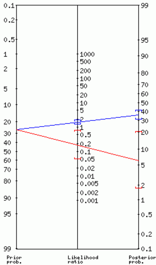
Fig. 3. Fagan nomogram
